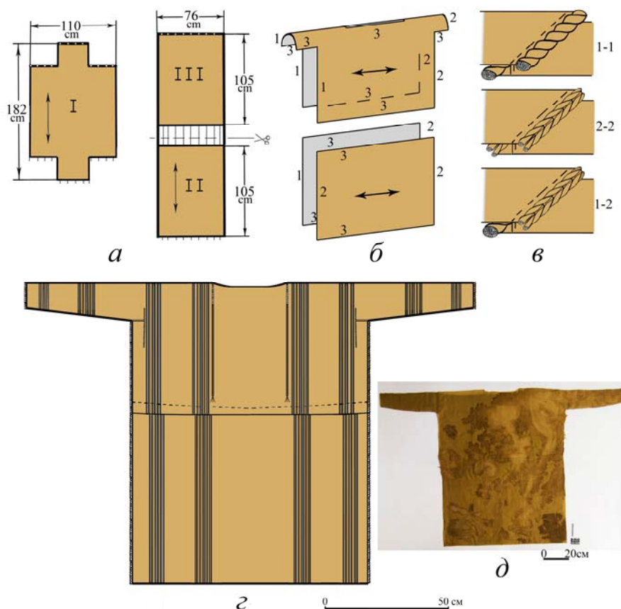
Рис. 4. Туника № 2008/0128/001/В (туника «В»): а — расположение частей туники «В» на ткацком станке; б — конструкция туники «В»; в — соединительные швы; г — графическая реконструкция туники «В»; д — общий вид туники «В» после реставрации (реставрационная группа под руководством Н.П. Синецкой).
