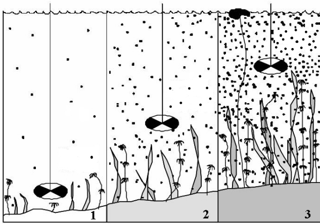
Рис. 3. Различные градации трофности и условного развития гидробионтов в водоёмах с различной прозрачностью воды (по [14]). Типы трофности: 1 — олиготрофные; 2 — мезотрофные; 3 — эвтрофные
