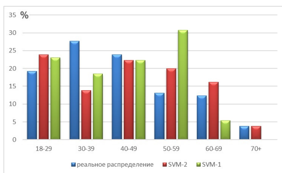
Рис. 3. Реальное распределение возрастных групп в тестовой выборке и варианты распределений, основанные на индивидуальных точечных оценках регрессионных моделей SVM-1 и SVM-2.
