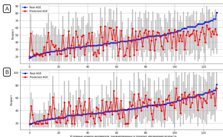
Рис. 2. Точечные оценки возраста и 95%-ные доверительные интервалы (серые столбики), рассчитанные для индивидов тестовой выборки по результатам применения регрессионных моделей SVM-1 (A) и SVM-2 (B).
