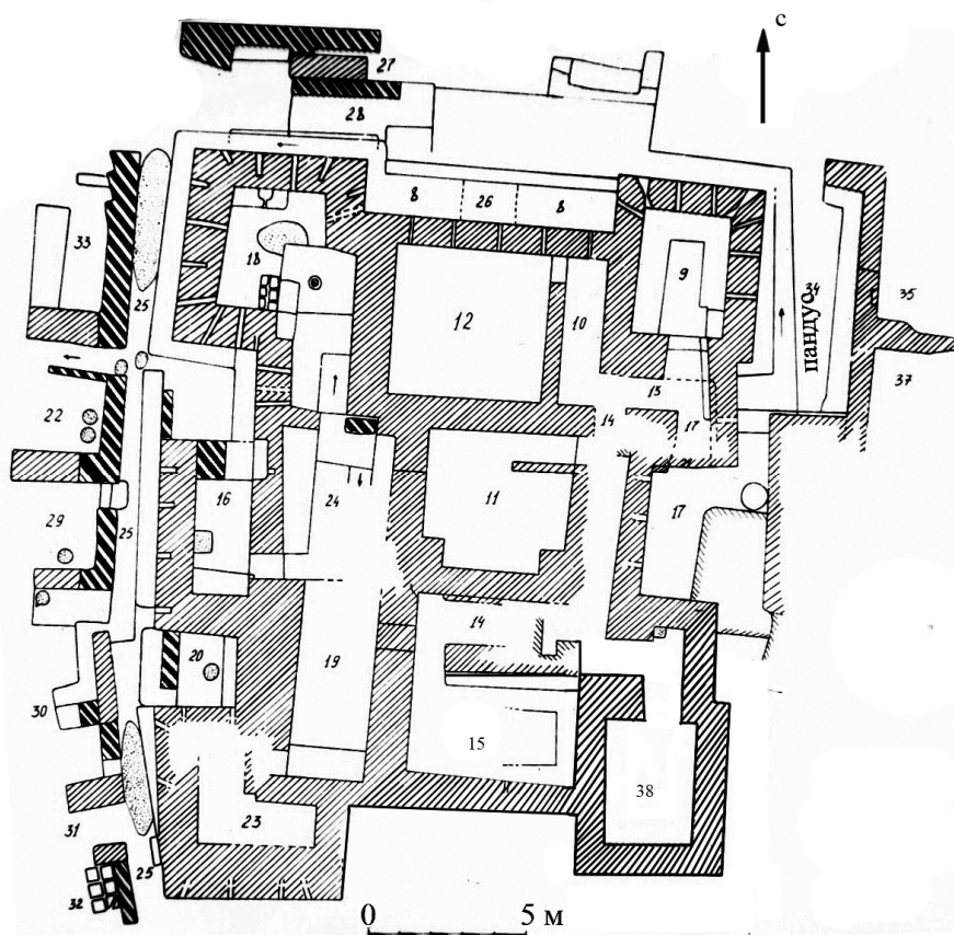
Рис. 2. План основного здания памятника Хантепа.
